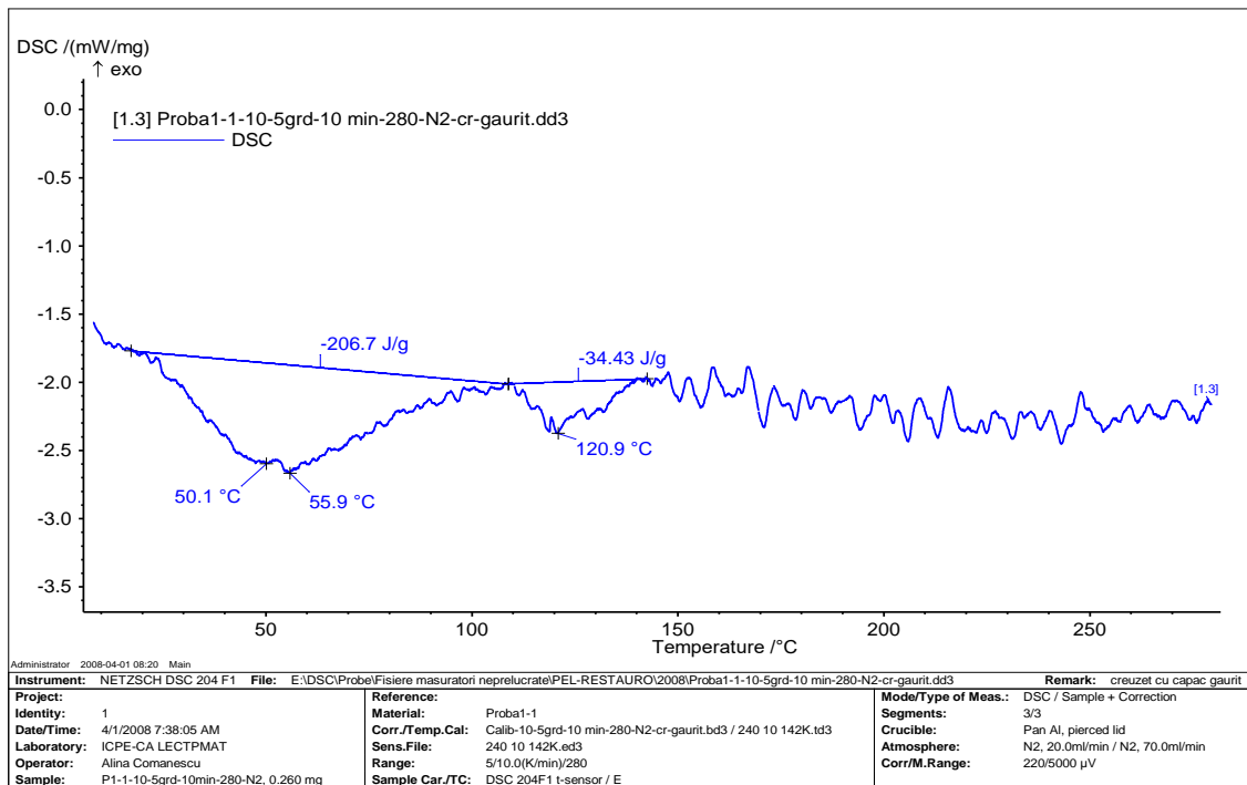
Fig. 1.1. Curba DSC pentru proba de piele P1-1
