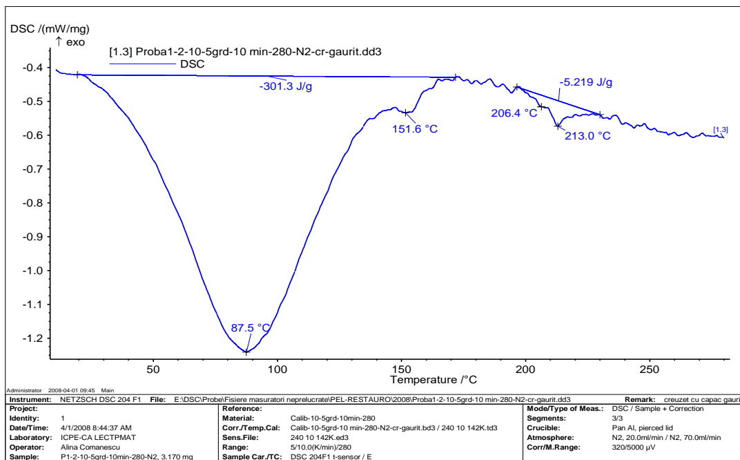
Fig. 1. 2. Curba DSC pentru proba de piele P1-2
