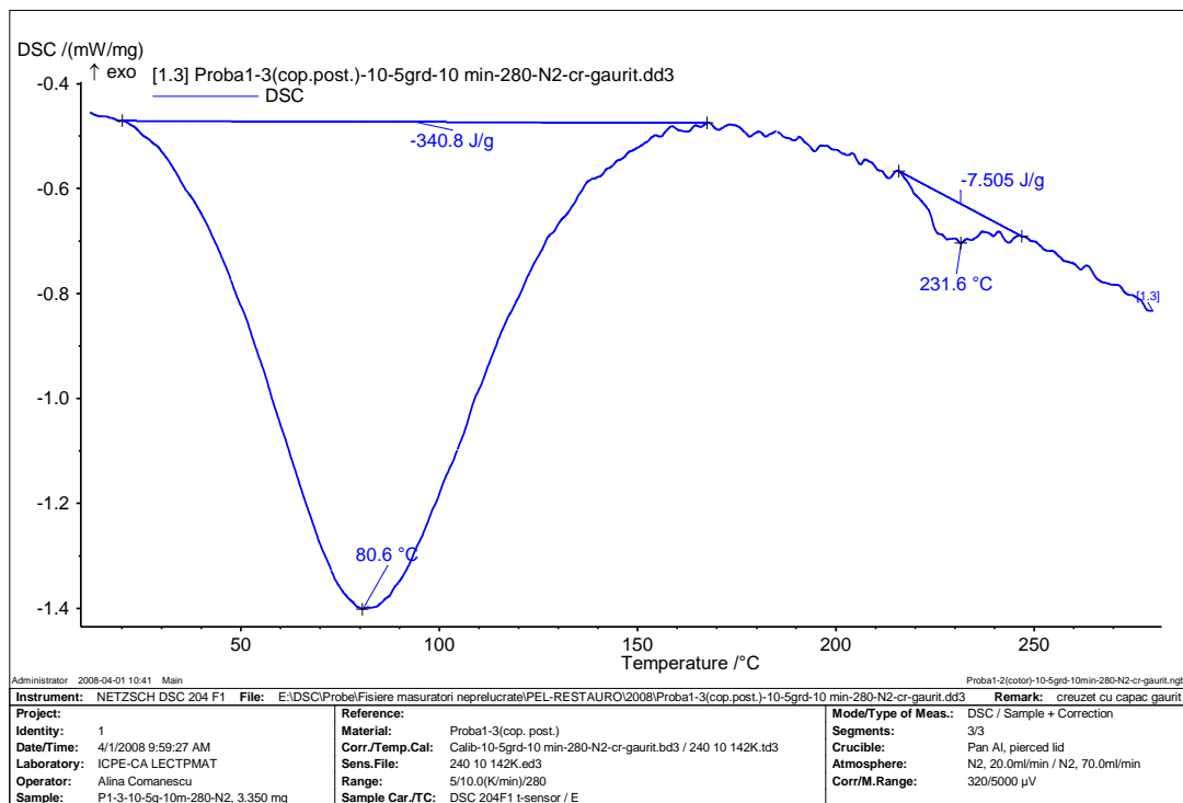
Fig. 1.3. Curba DSC pentru proba de piele P1-3
